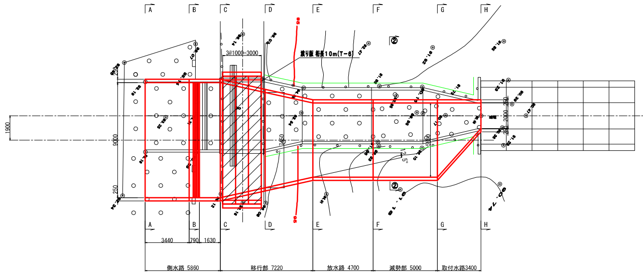
平面图
