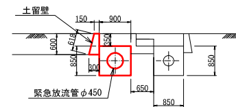
②-②断面
