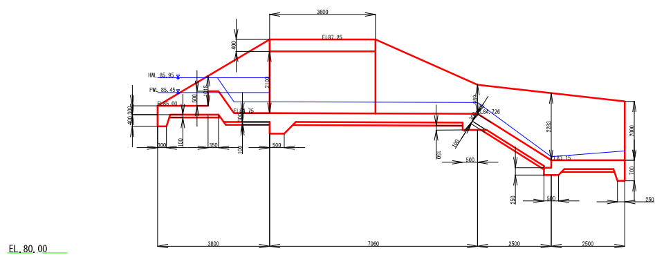
縦断図
