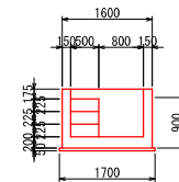
G—G断面
