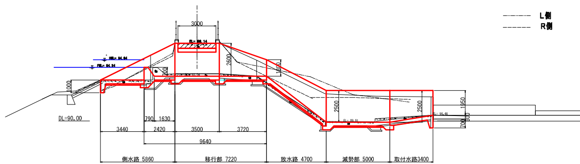
縦断面図
