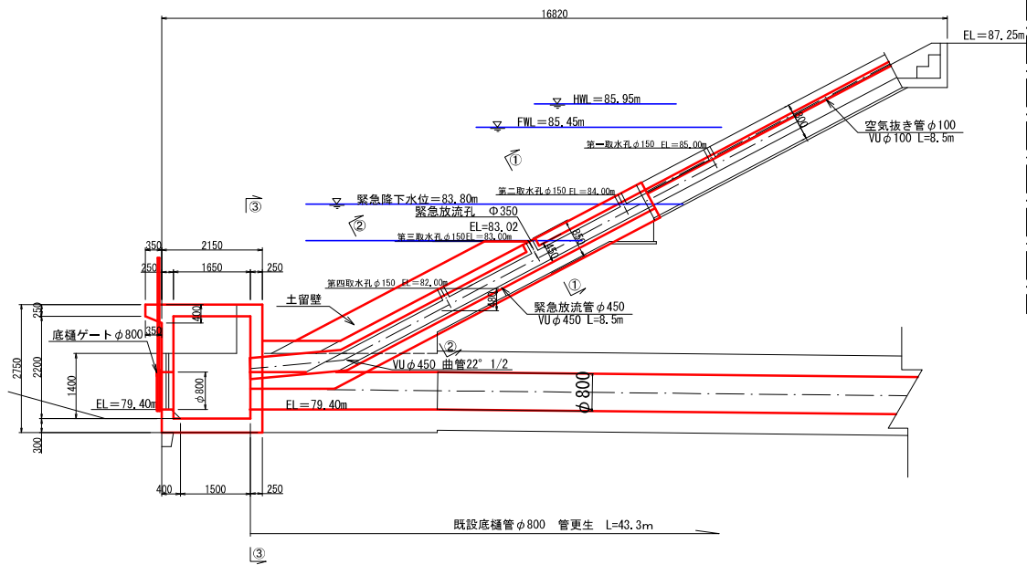
縦断図
