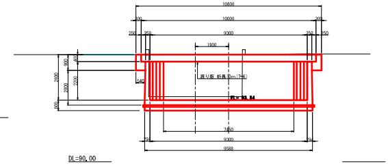
C-C (+) 断面图
