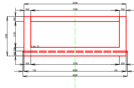
C-C (+) 断面图
