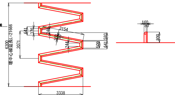
ラビリンス堰 詳細図
