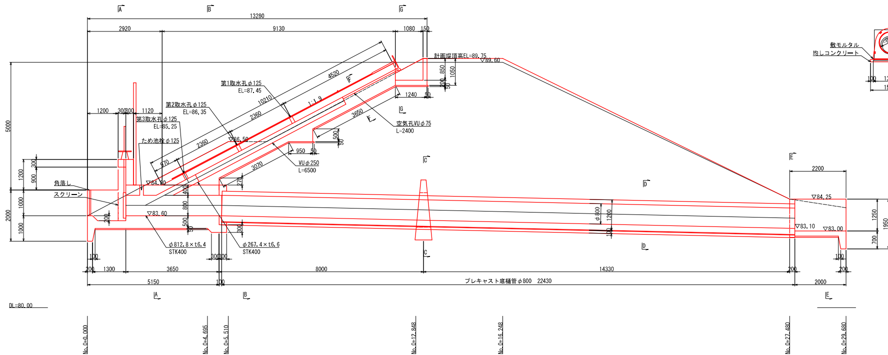
プレキャスト底樋横断面図
