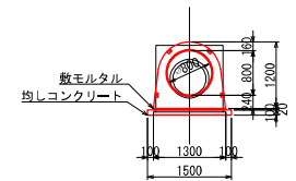
プレキャスト底樋横断面図
