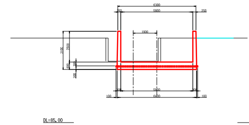
F-F断面图
