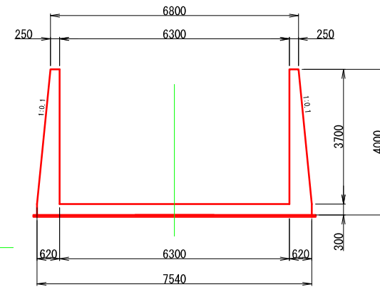
E-E断面
