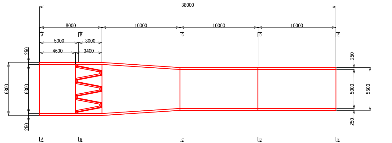
平面図
