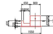
F-F断面
