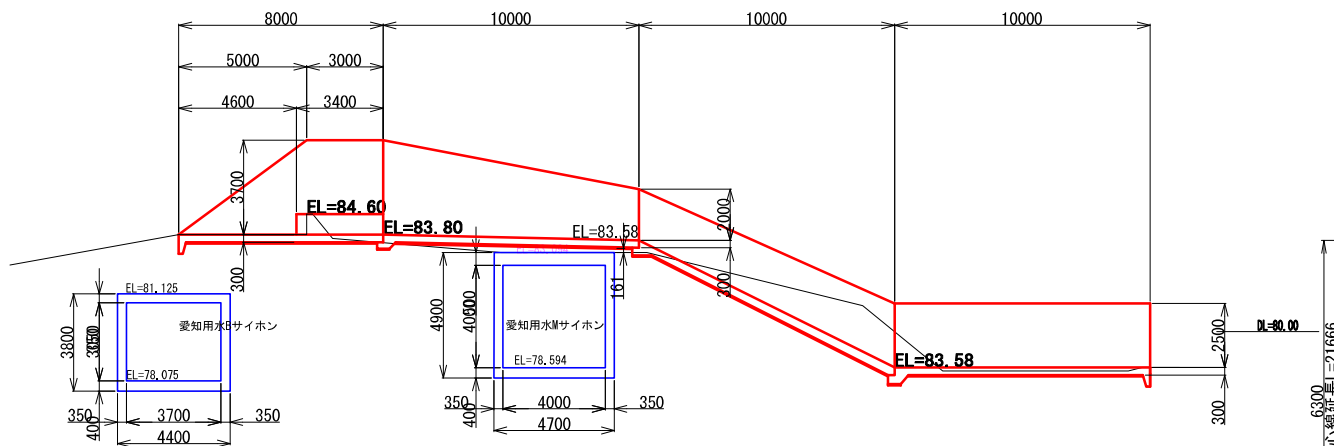
縦断面図
