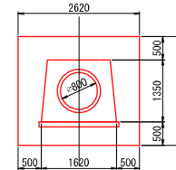
C-C断面
