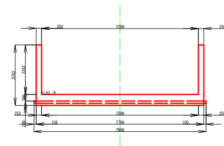
E-E断面图
