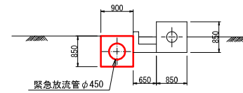
①—①断面
