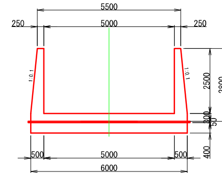
ラビリンス堰 詳細図
