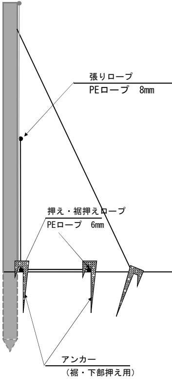
【側面図】
