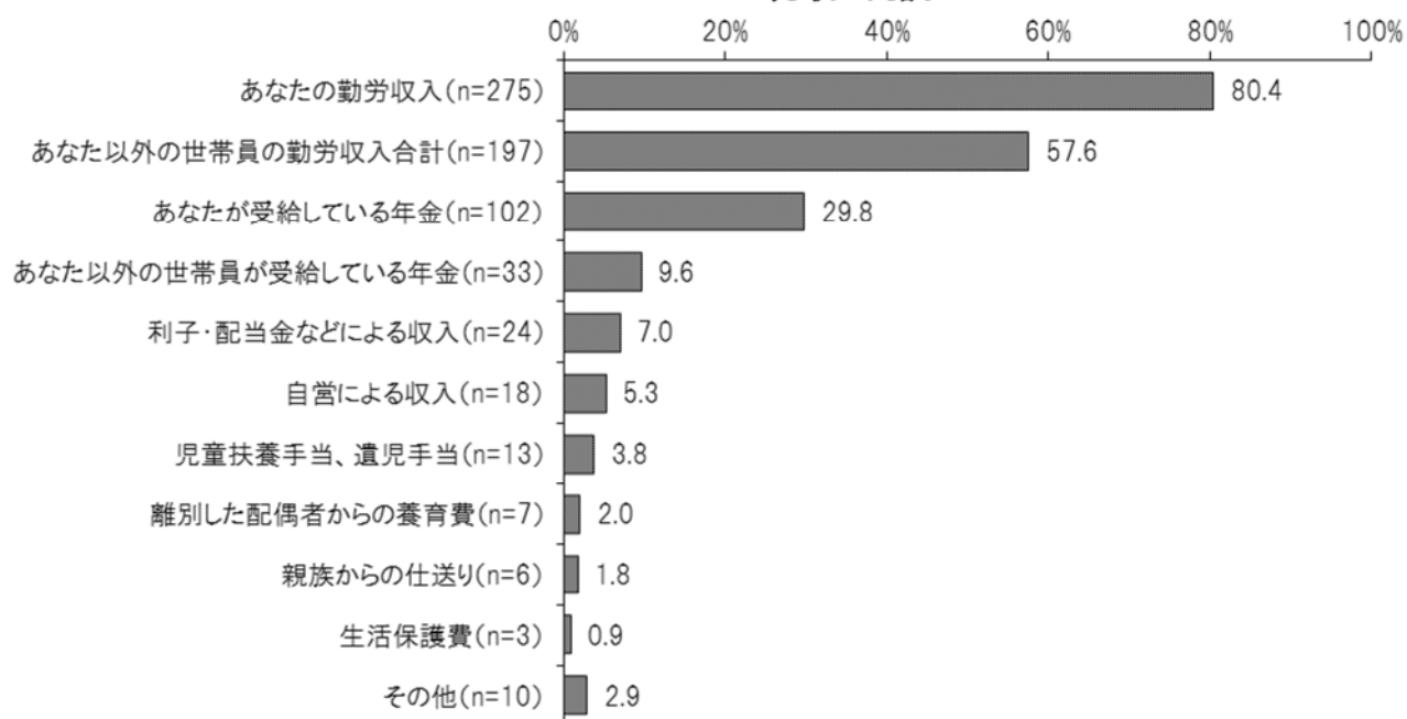
月収の内訳
