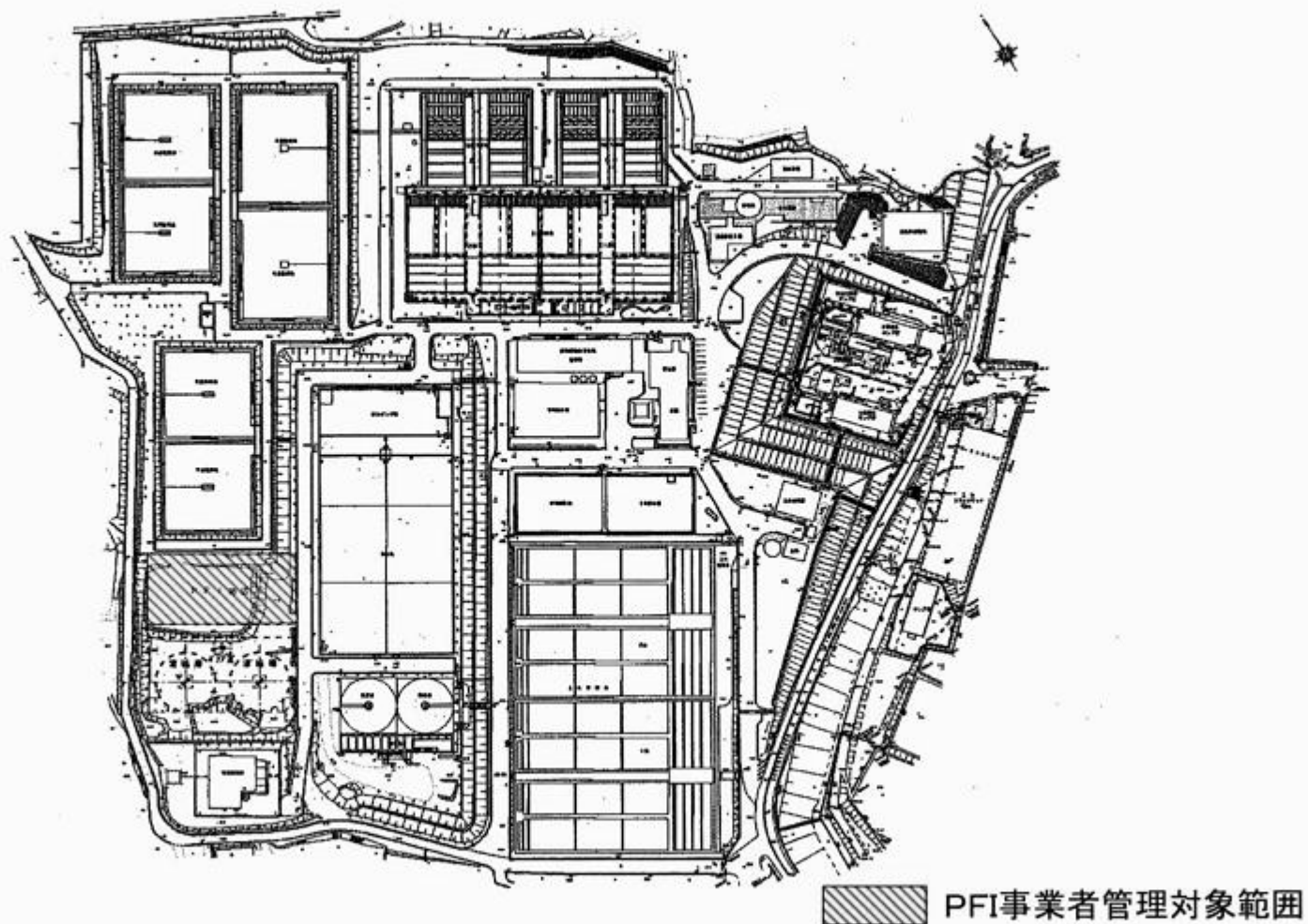
知多浄水場 平面図
