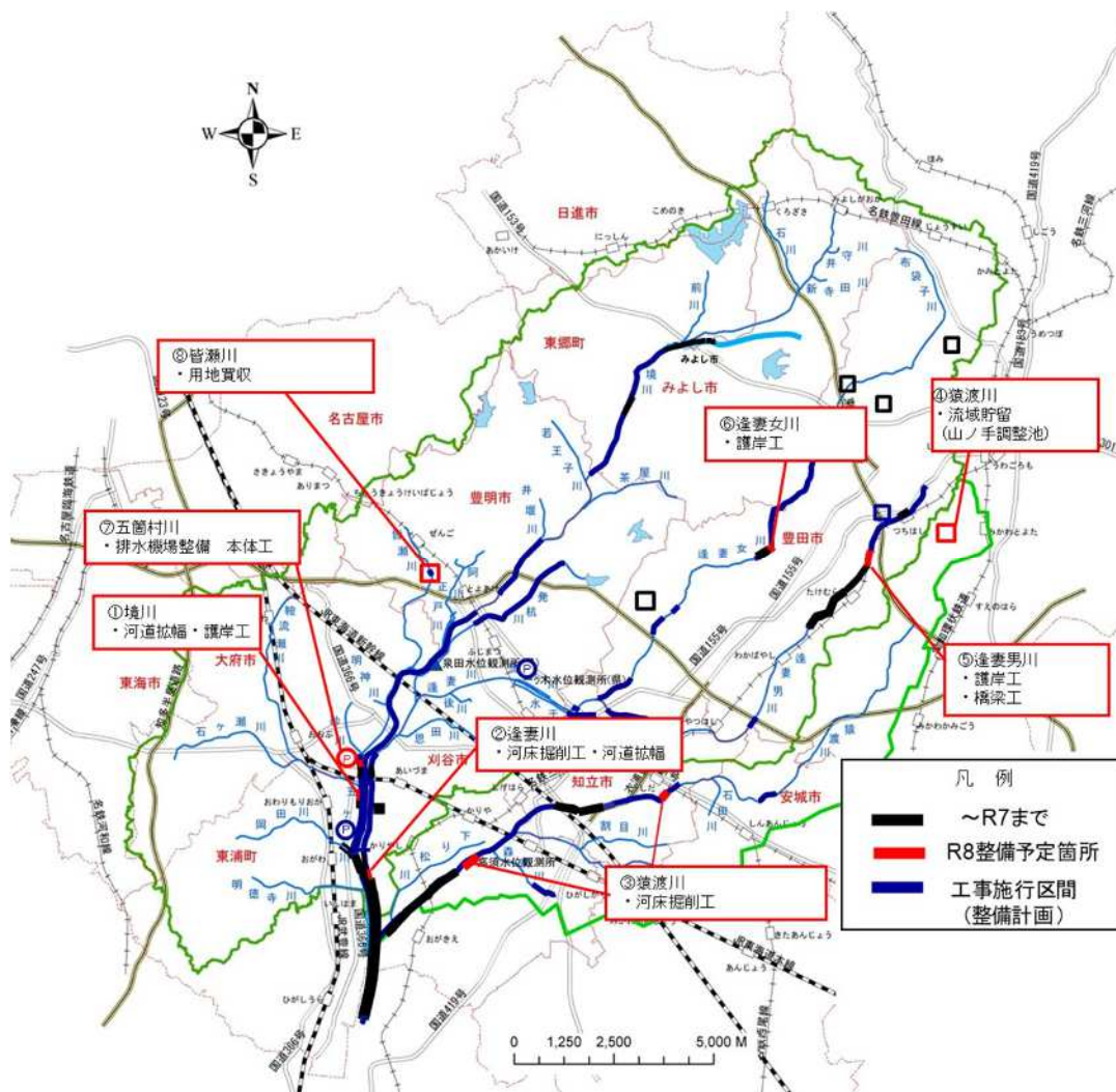
⑥ 逢妻女川：護岸工実施予定 (松竹橋上流)
