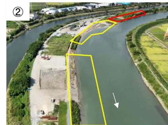
② 逢妻川：河道拡幅実施予定 (JR東海道本線付近)
