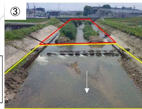
③ 猿渡川：河床掘削実施予定 (八ツ田橋下流)
