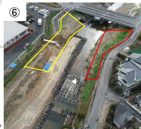
⑥ 逢妻女川：護岸工実施予定 (松竹橋上流)
