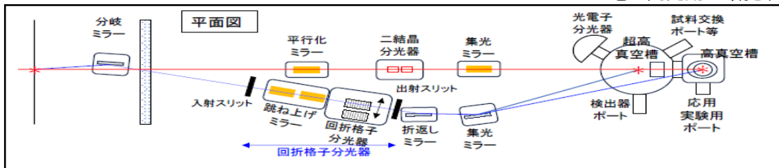
電池開発用BL概念図
