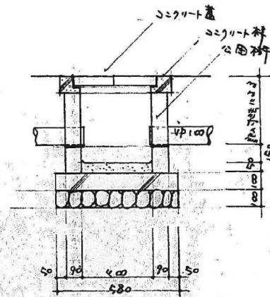
雨水管詳細図
