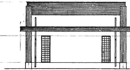
③ 正面図 1/100
