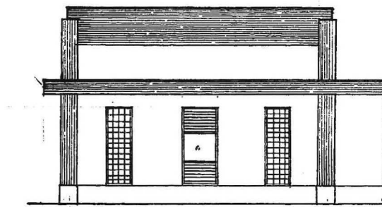
④ 正面図 1/100
