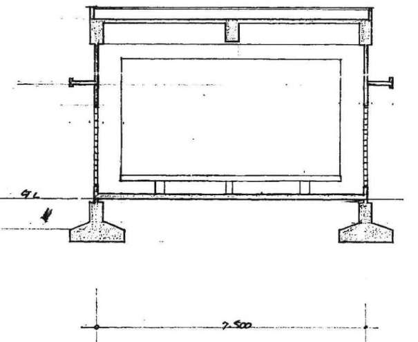
A-A 断面図
