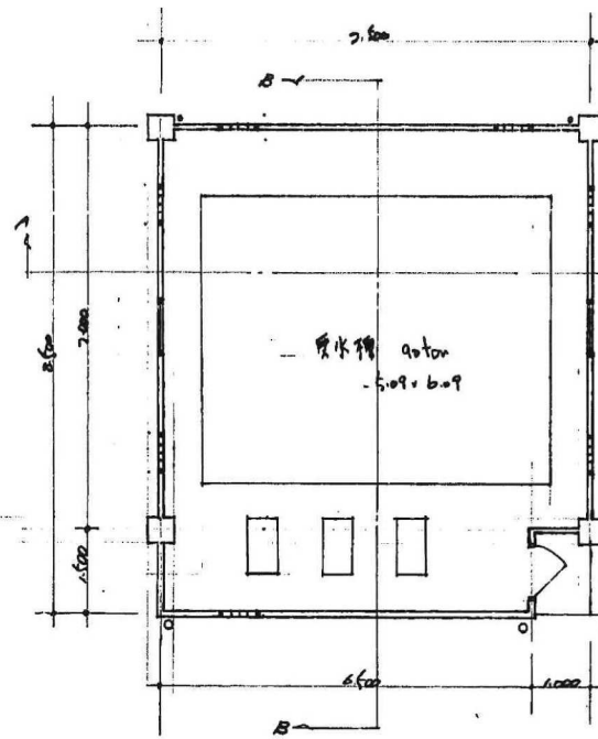
平面図 1/100
