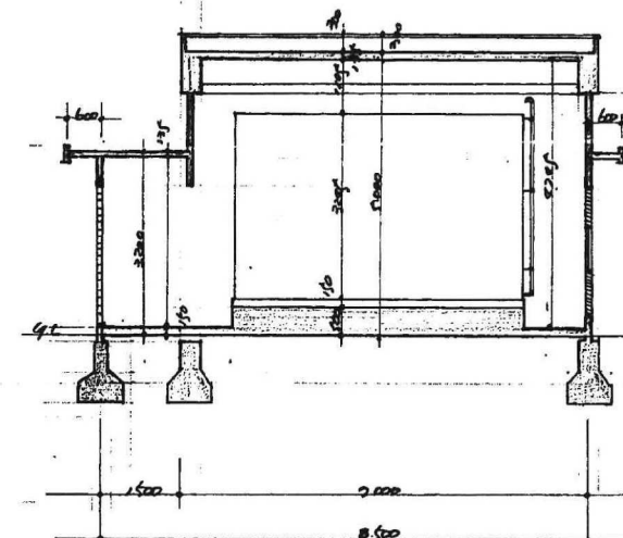
B-B 断面図
