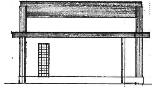
① 正面図 1/100
