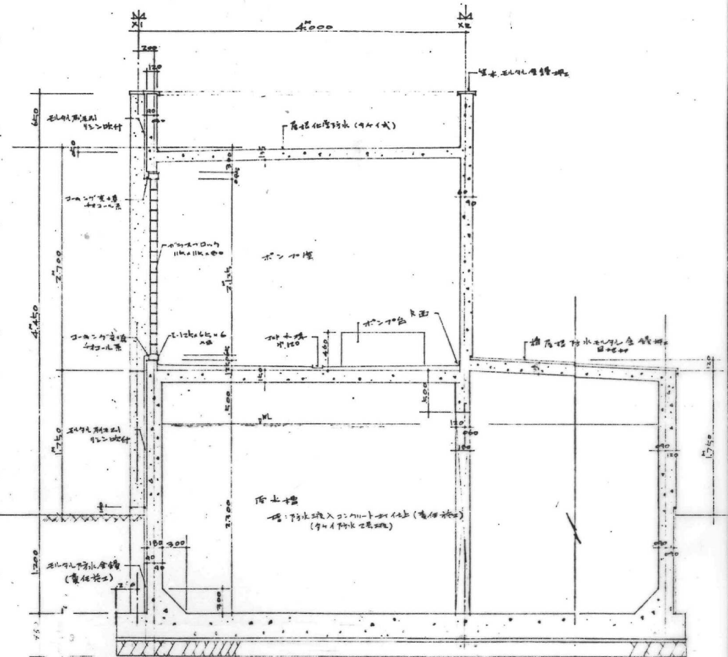
断面図 1:30
