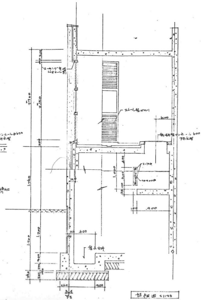
コンクリート壁詳細図 1:30
