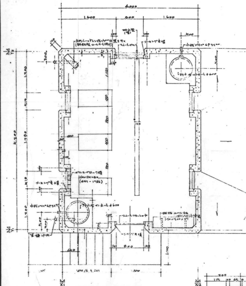
平面詳細図 1:30
