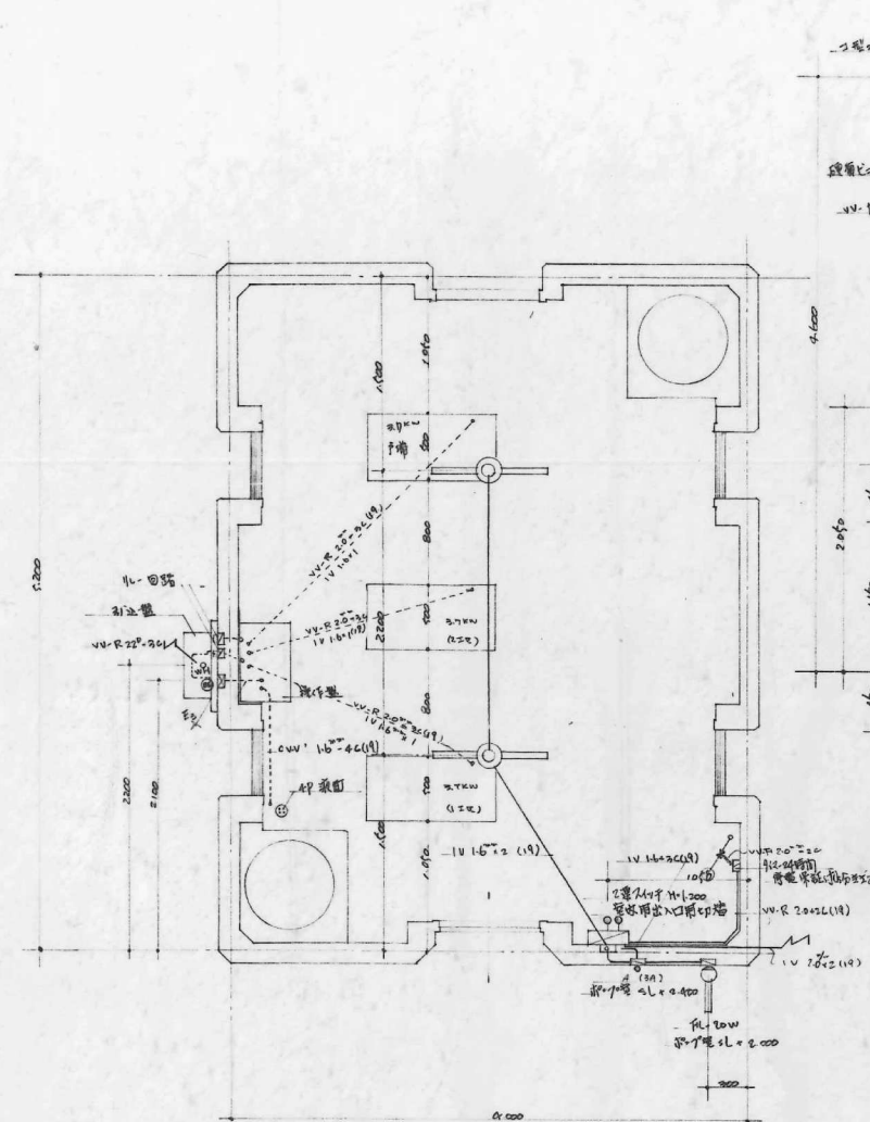
配線器具取付図 V20
