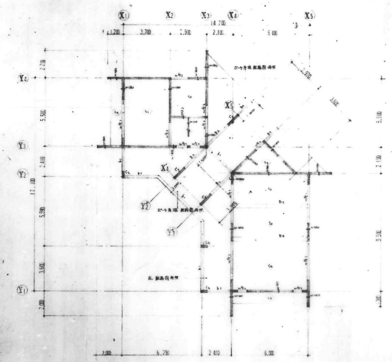
第3号会所 壁根伏図 1/100
