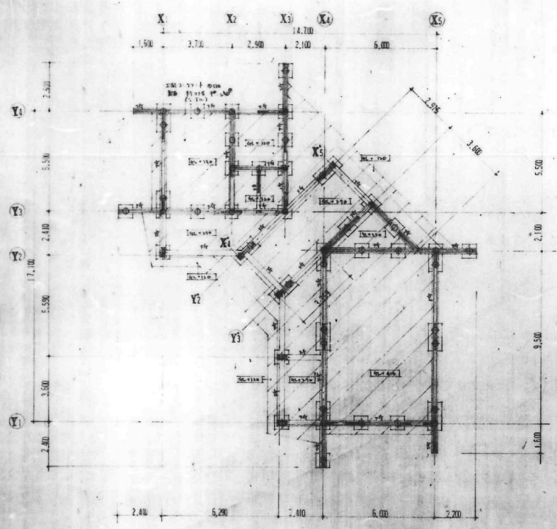
第3号会所 基礎伏図 1/100
