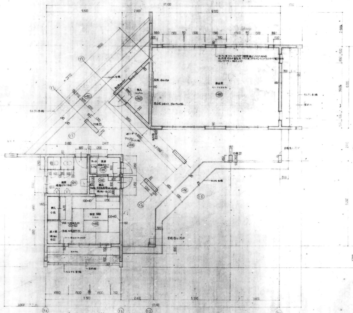
第3集会所平面詳細図 1/50
