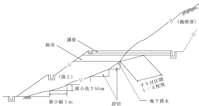
図 1 - 2 盛土基礎地盤の段切
