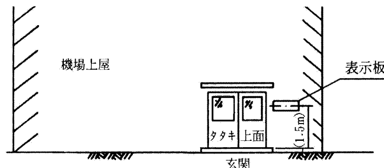
図3-2 排水機場の銘板及び標示板の取付け場所
