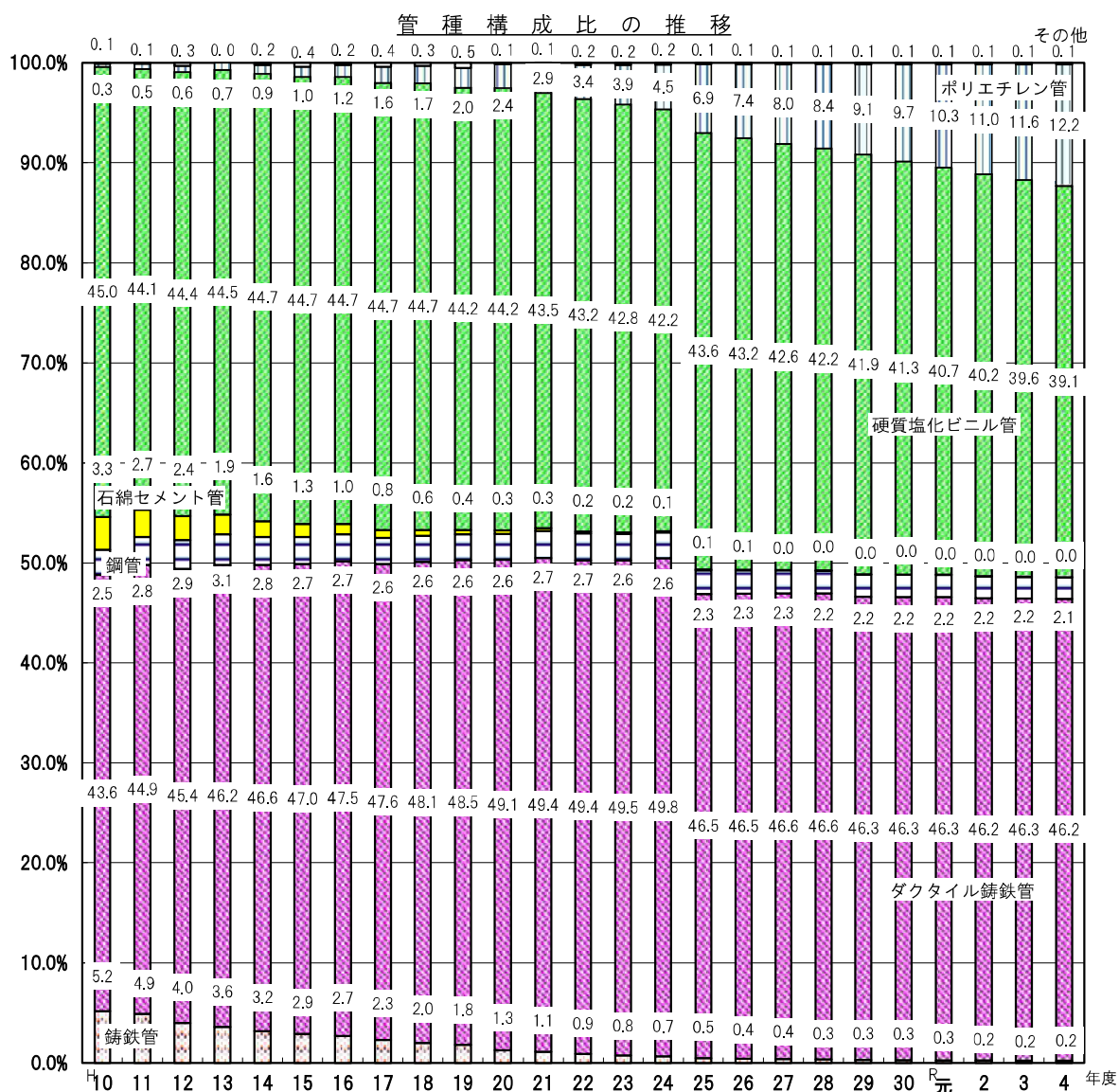
図一8 管路延長及び管種構成比の推移
