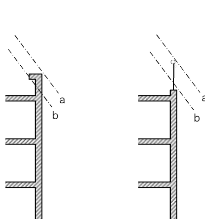
【図4】パラペット
