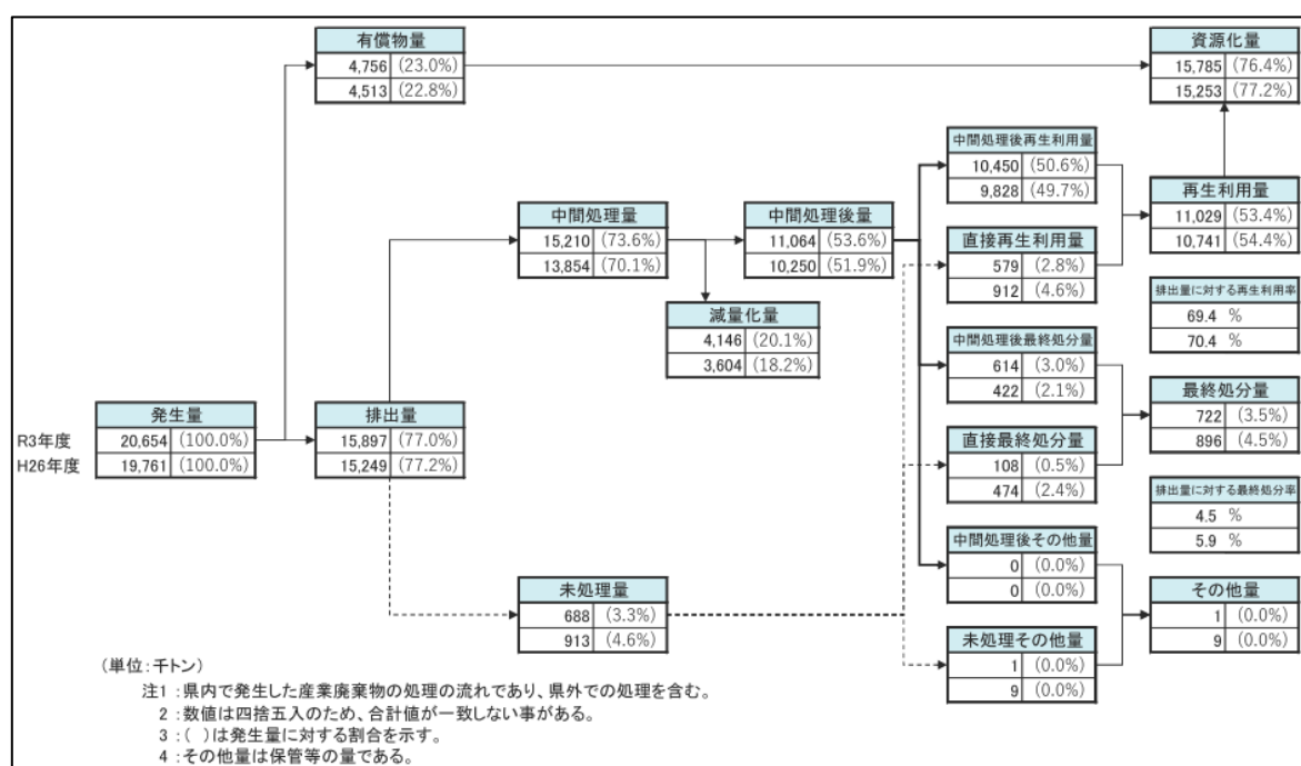
図 3.2-12 産業廃棄物の処理の流れ
