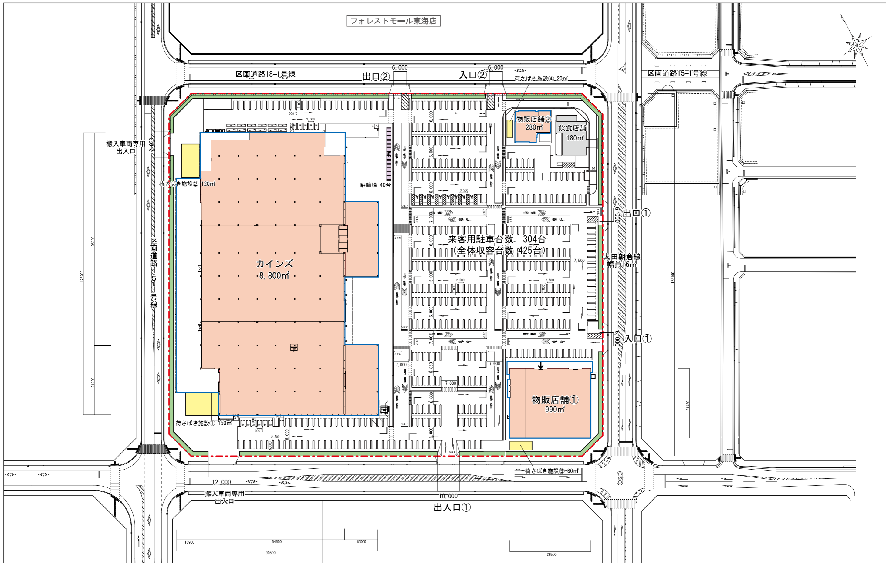
図面 3 建物配置図 (S=1/1,000)
