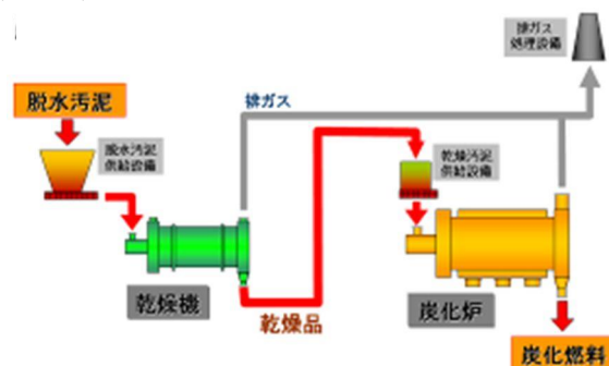
衣浦東部浄化センター 污泥処理フロー
