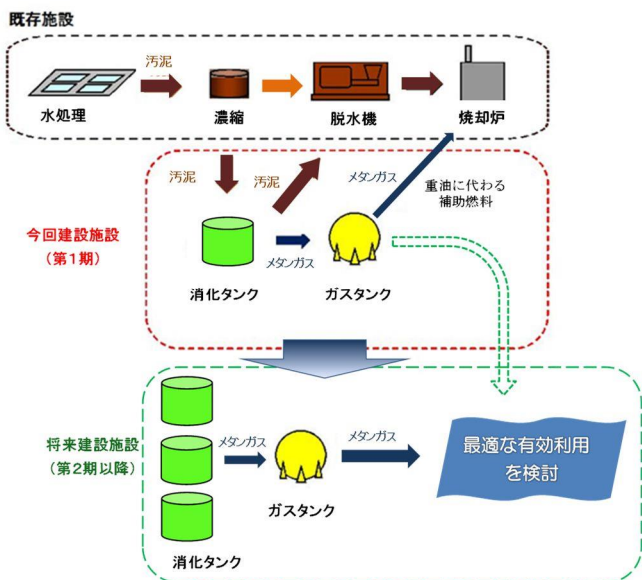
污泥処理フロー
