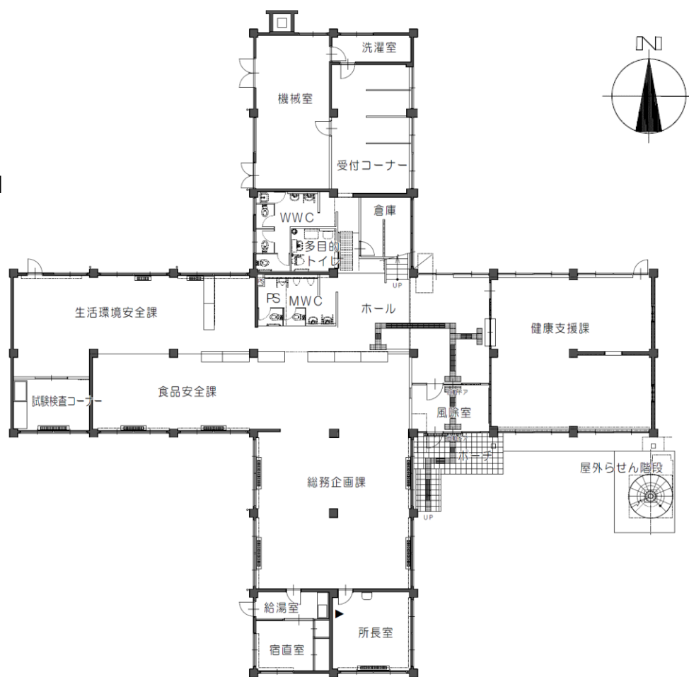
一階平面図
