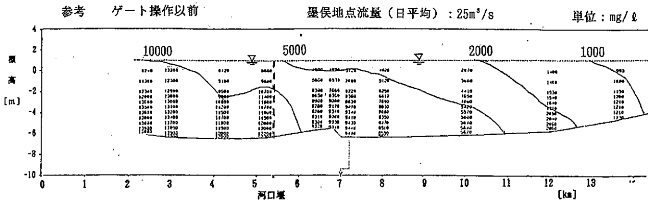
図-7-1-2-(7) 水質詳細調査 塩化物イオン濃度河川縦断面図 (7月12日 8時 満潮)
