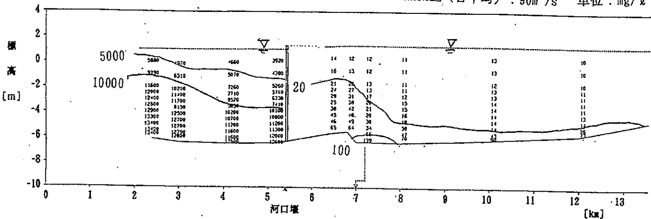
図-7-1-2-(3) 水質詳細調査 塩化物イオン濃度河川縦断面図（9月22日8時 満潮）
