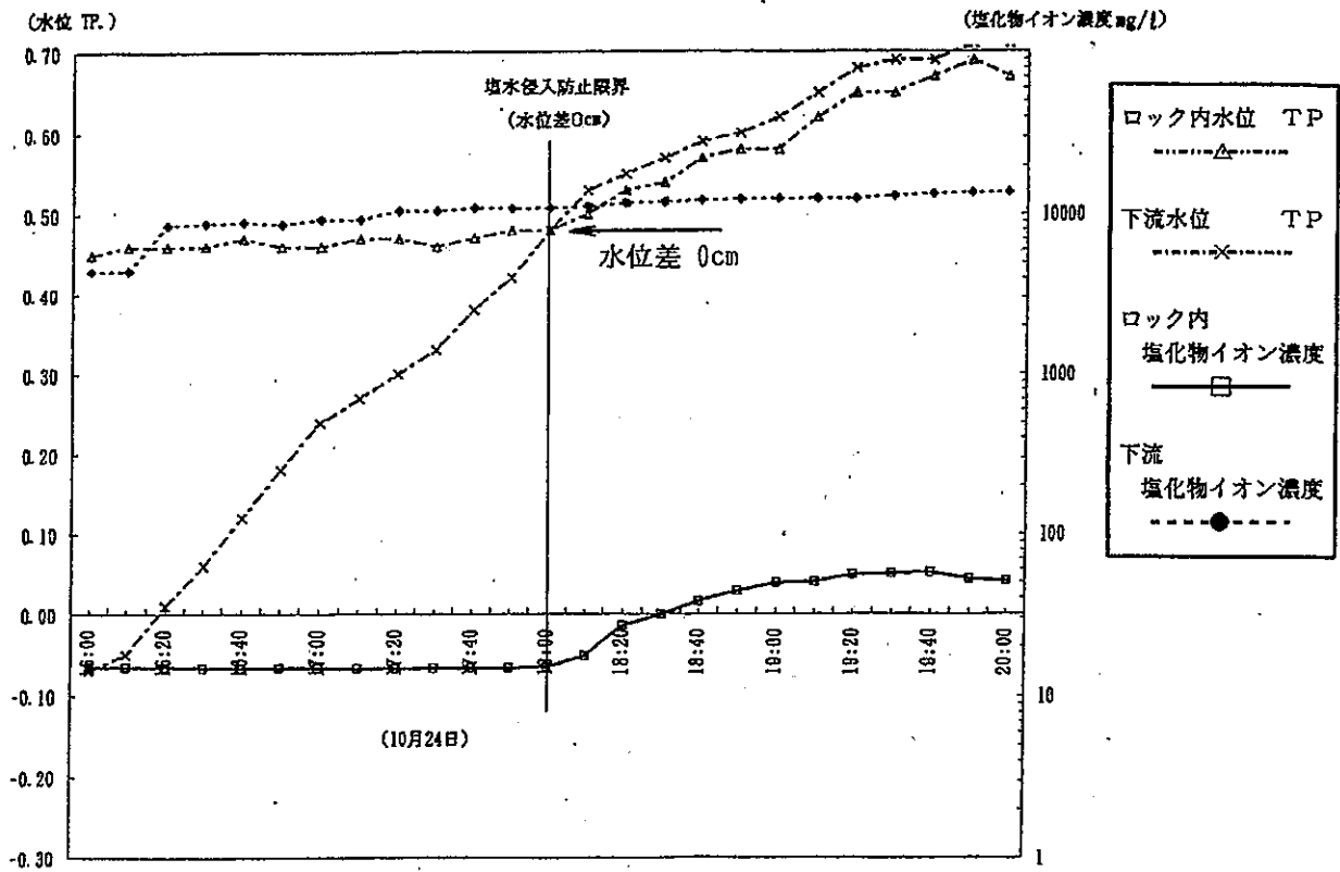
図-7-1-9-(3) オーバーフロー時の塩水侵入状況図 (一門あたり流量約12m 3 /s)
