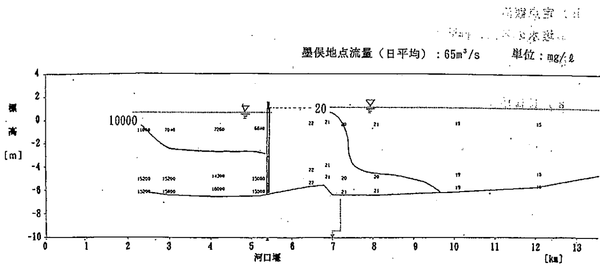
図-7-1-2-(6) 水質詳細調査 塩化物イオン濃度河川縦断面図 (10月24日 8時 満潮)
