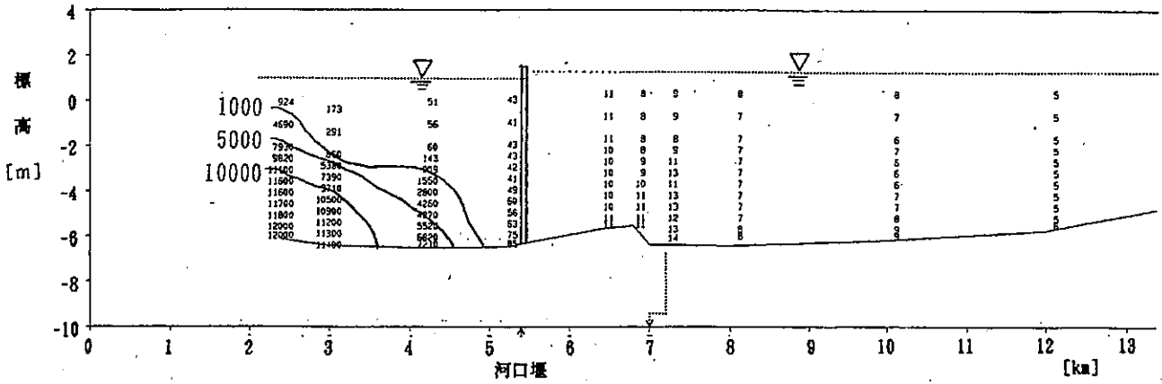
図-7-1-2-(2) 水質詳細調査 塩化物イオン濃度河川縦断面図（9月20日7時 満潮）
