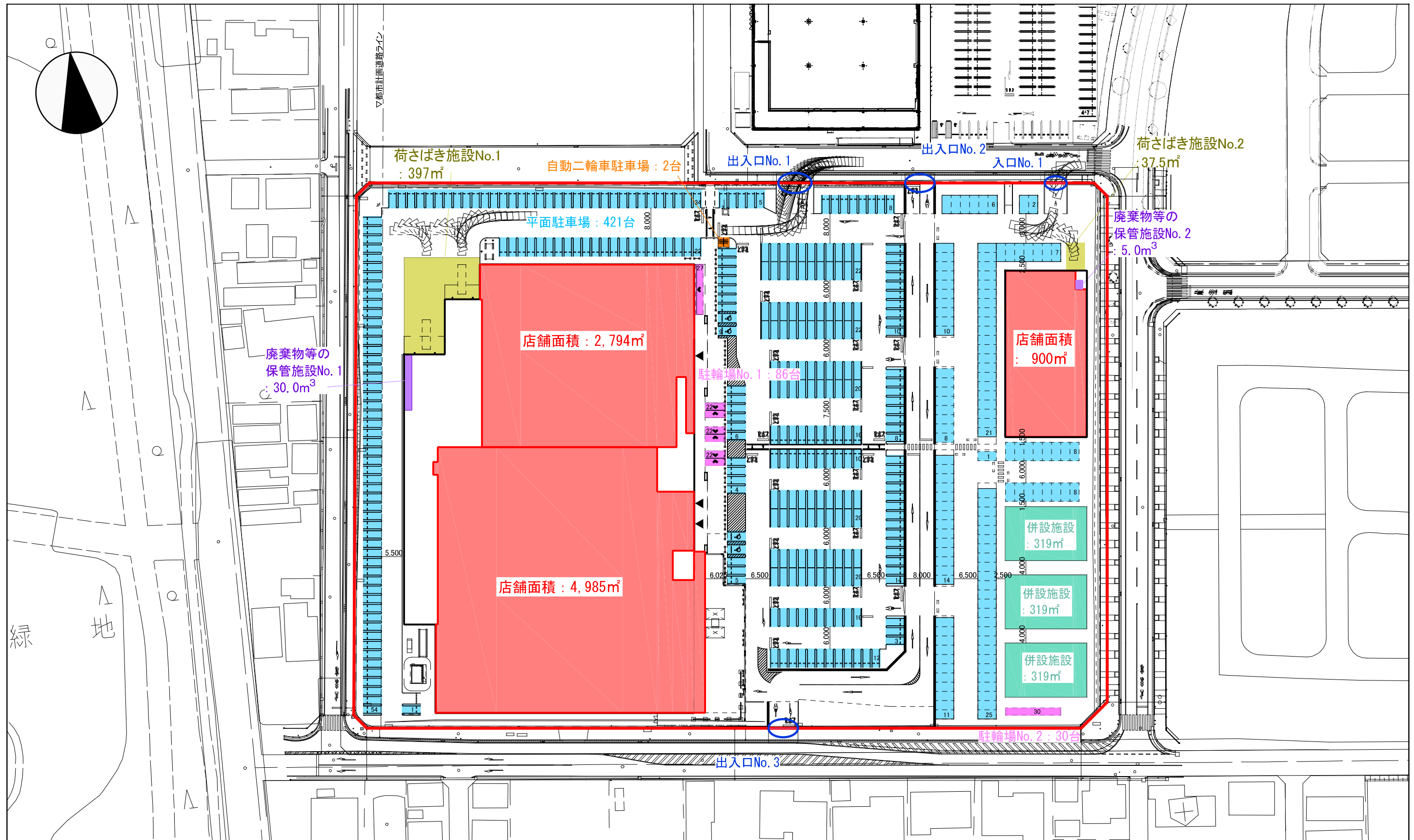
図面3 建物配置図兼 1階平面図 (S=1/1,000)
