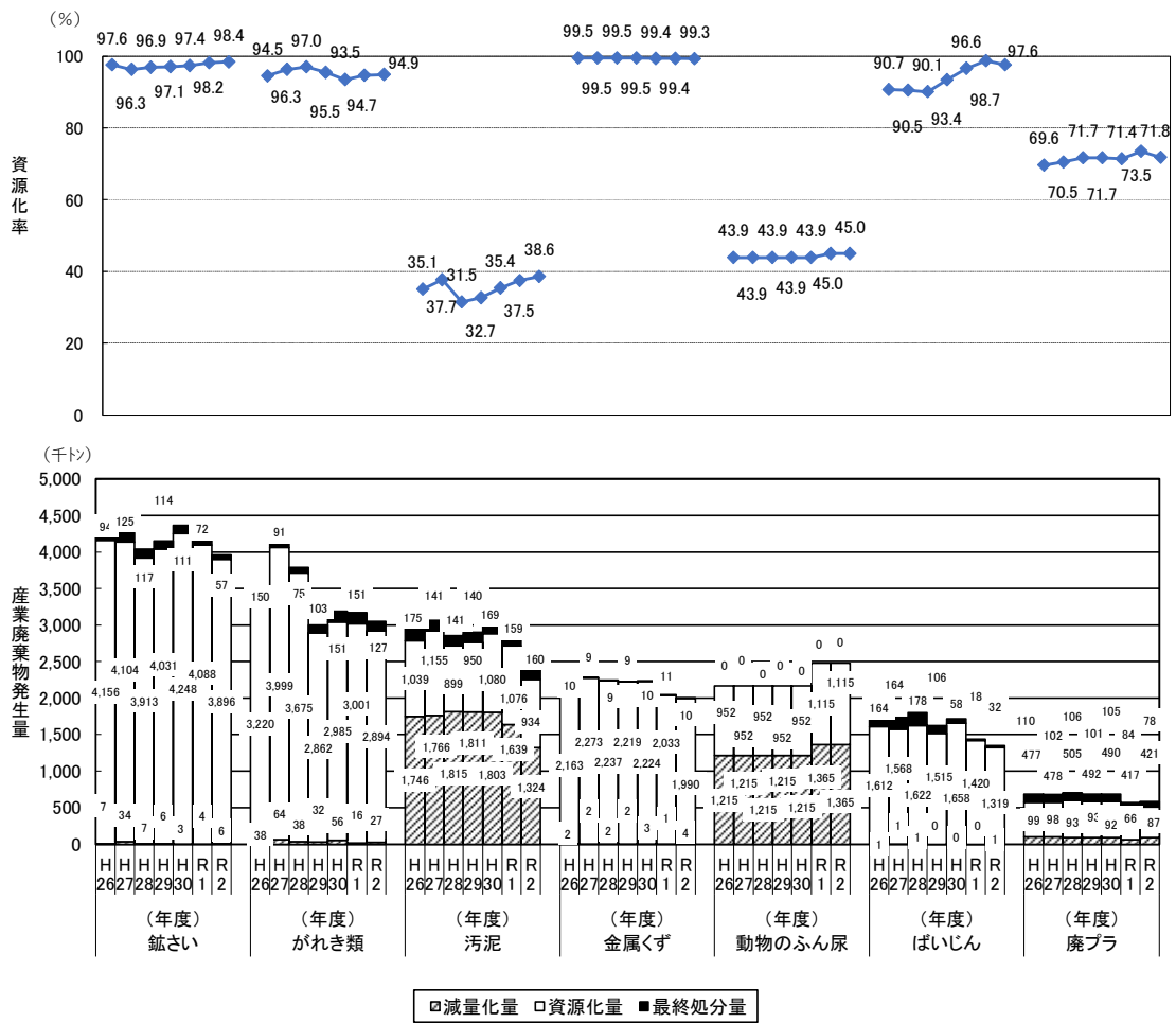
図 2-11 産業廃棄物の処理状況の経年変化
