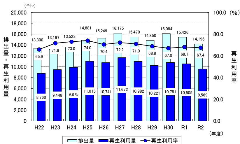
図 2-14 再生利用率の推移
