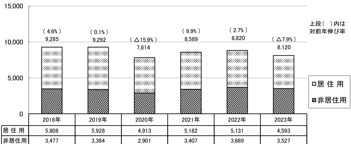
(千㎡) 建築物の着工床面積の推移(2018年以降)
