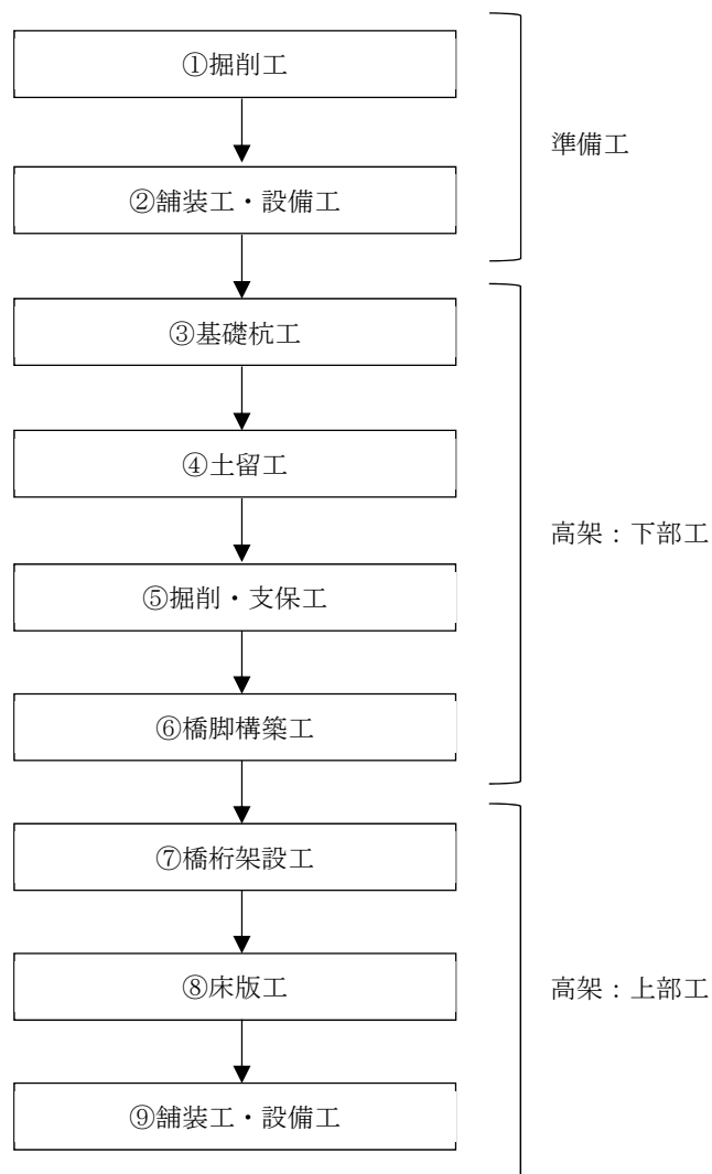
図 3-6(1) 施工手順
