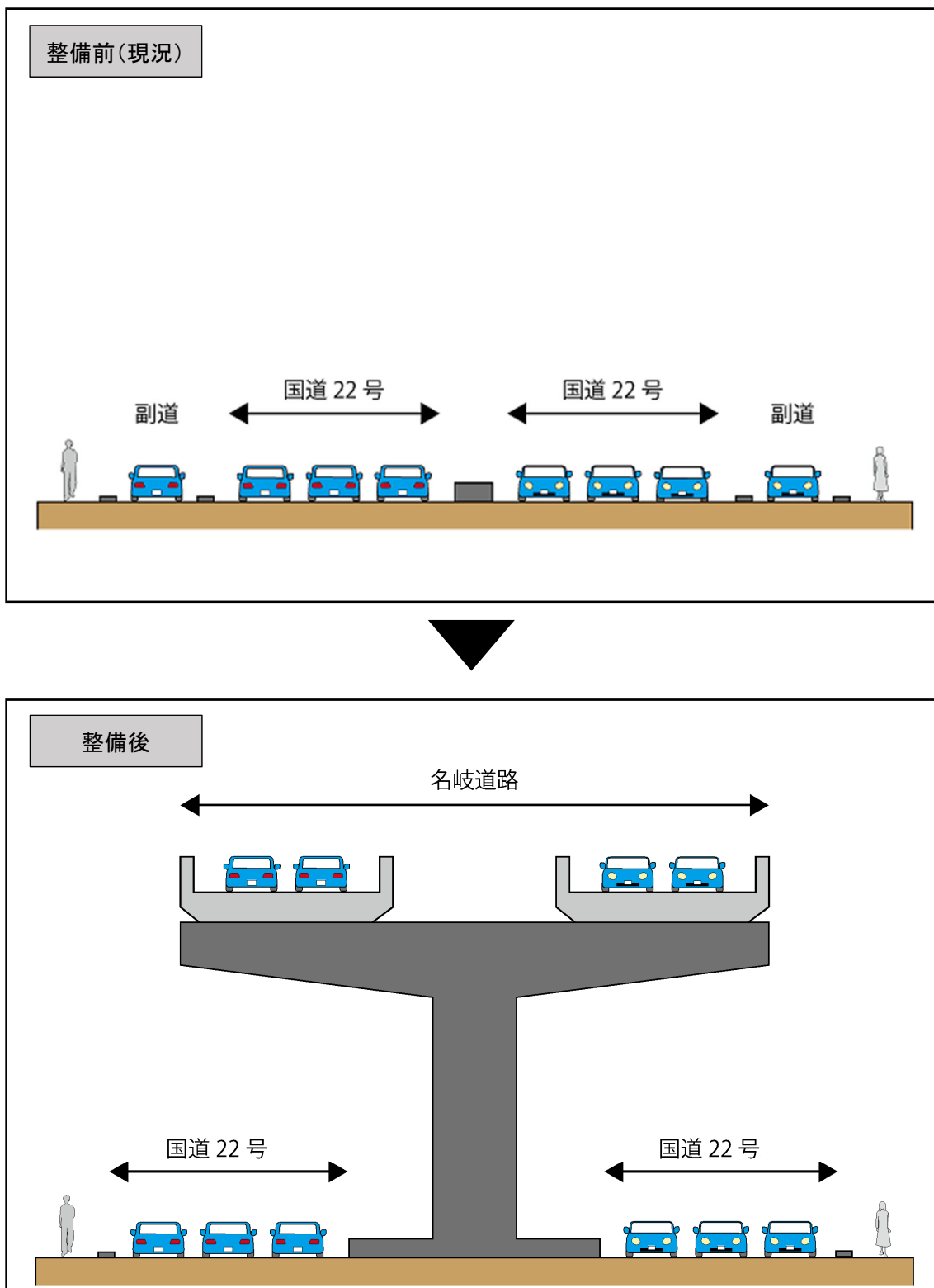
図 3-5 道路構造図（標準断面図）
