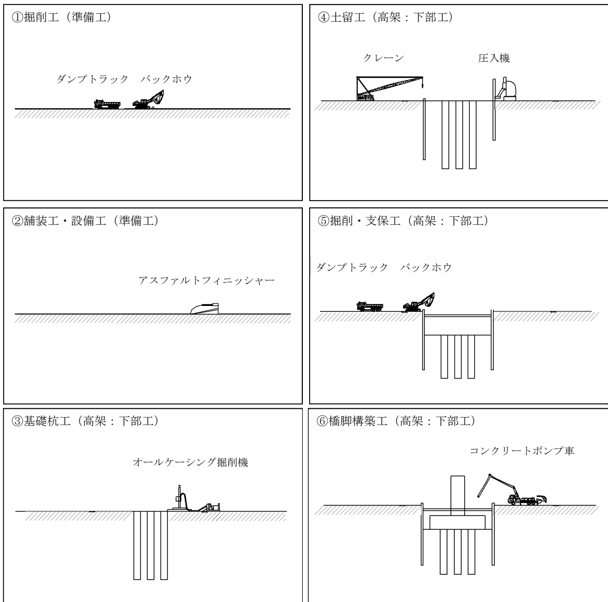
図 3-6(2) 施工手順
