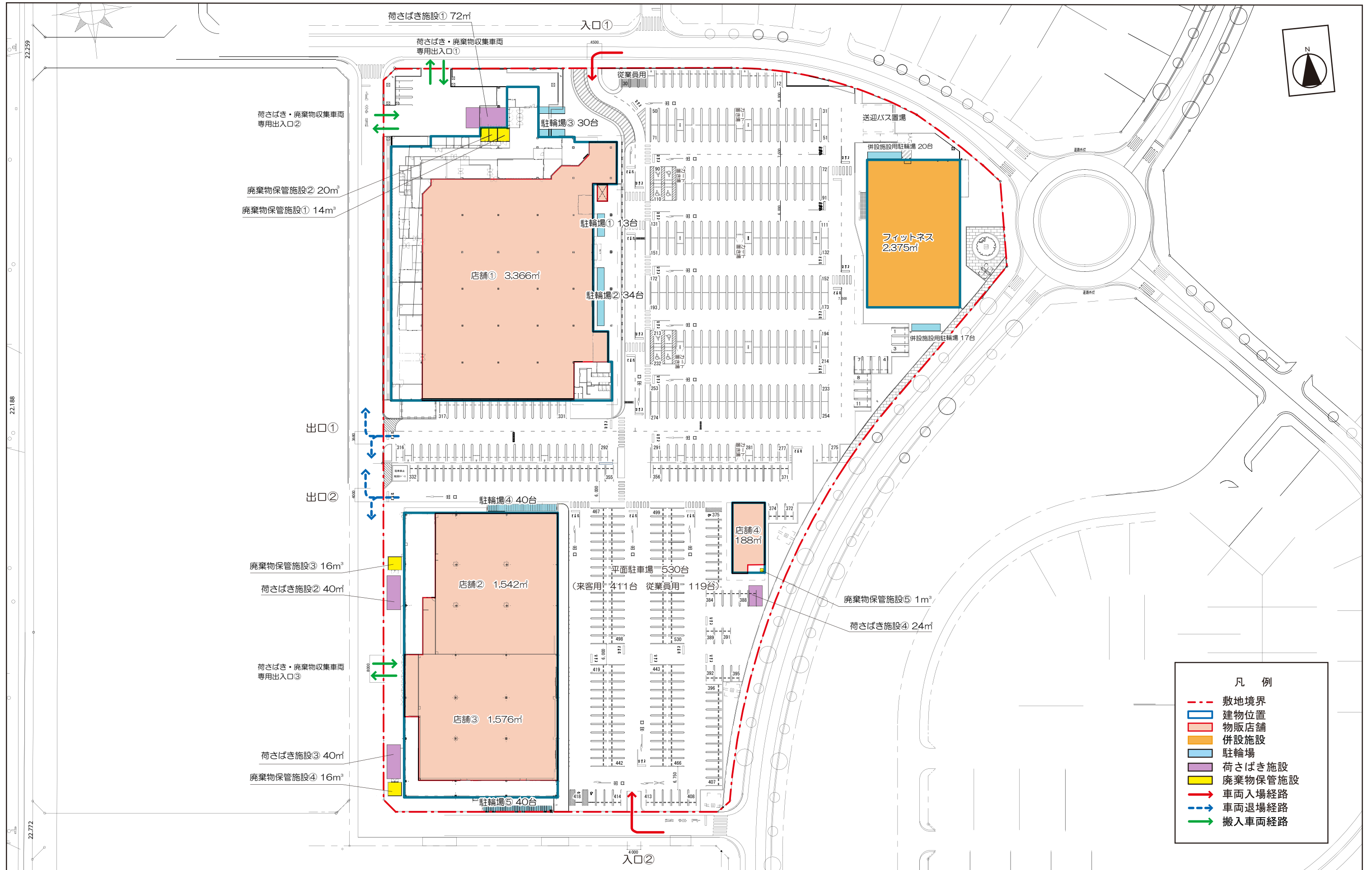
図面4 変更後建物配置図兼1階平面図(S=1/1,000)
