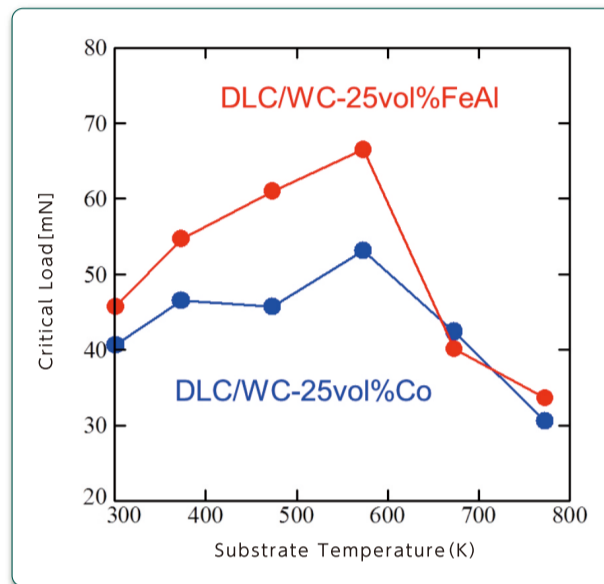
図1 DLC膜と基材との密着性
