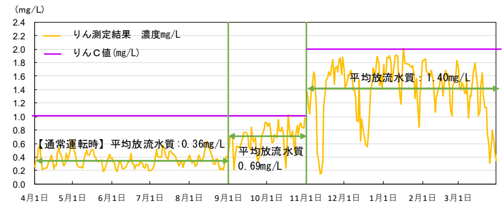
図4 豊川浄化センターにおける 2022 年度社会実験による放流水のリン濃度
