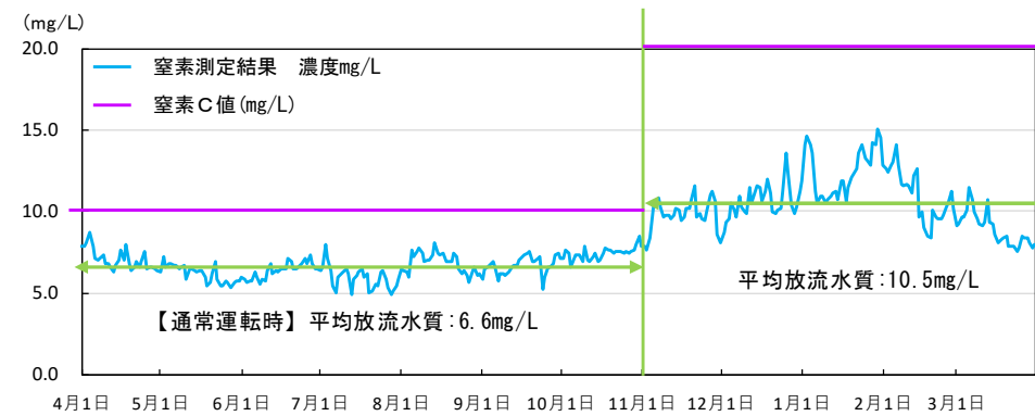
図1 矢作川浄化センターにおける 2022 年度社会実験による放流水の窒素濃度
