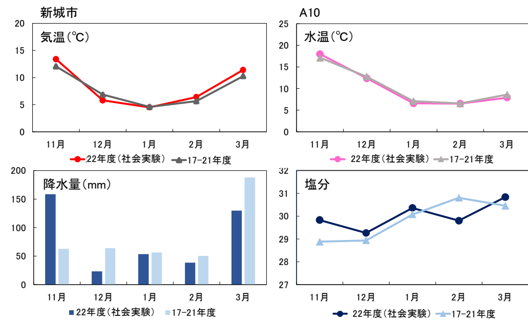
図 18 豊川地区の月平均気温・降水量(新城市)及び水温・塩分(A-10)の推移
