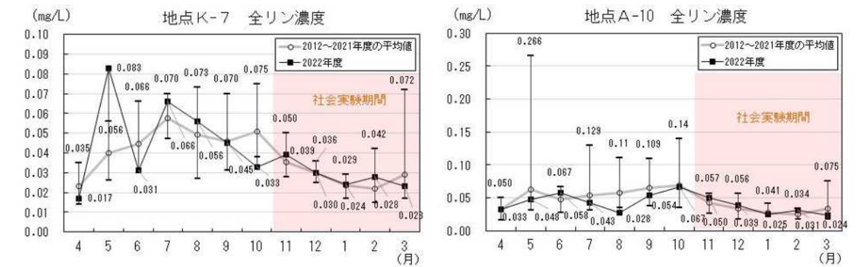
図7 2022年度の地点K-7・A-10の月別全リン濃度及び過去10年間の平均値と最大値・最小値
