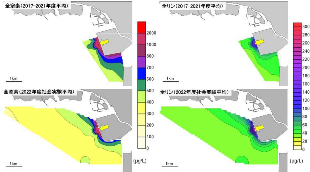
図 11 豊川地区の全窒素、全リン濃度分布(11~3月平均)
