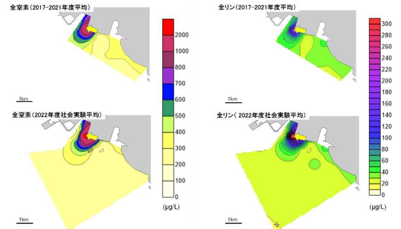
図 10 矢作川地区の全窒素、全リン濃度分布 (11~3 月平均)
