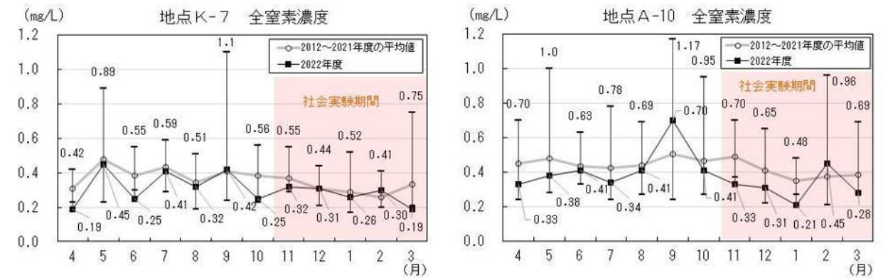
図6 2022年度の地点K-7・A-10の月別全窒素濃度及び過去10年間の平均値と最大値・最小値
