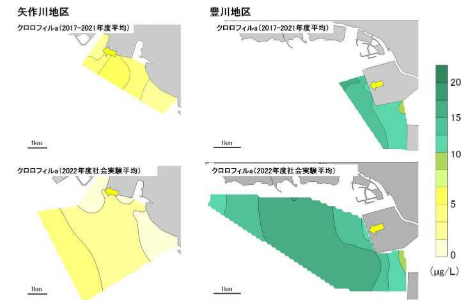
図 14 矢作川地区(左上、左下)、豊川地区(右上、右下)におけるクロロフィル a 濃度の分布(11~3月平均)
