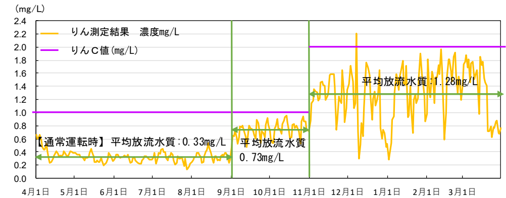
図3 矢作川浄化センターにおける 2022 年度社会実験による放流水のリン濃度
