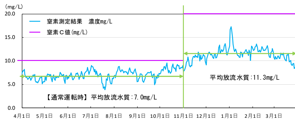
図2 豊川浄化センターにおける 2022 年度社会実験による放流水の窒素濃度
