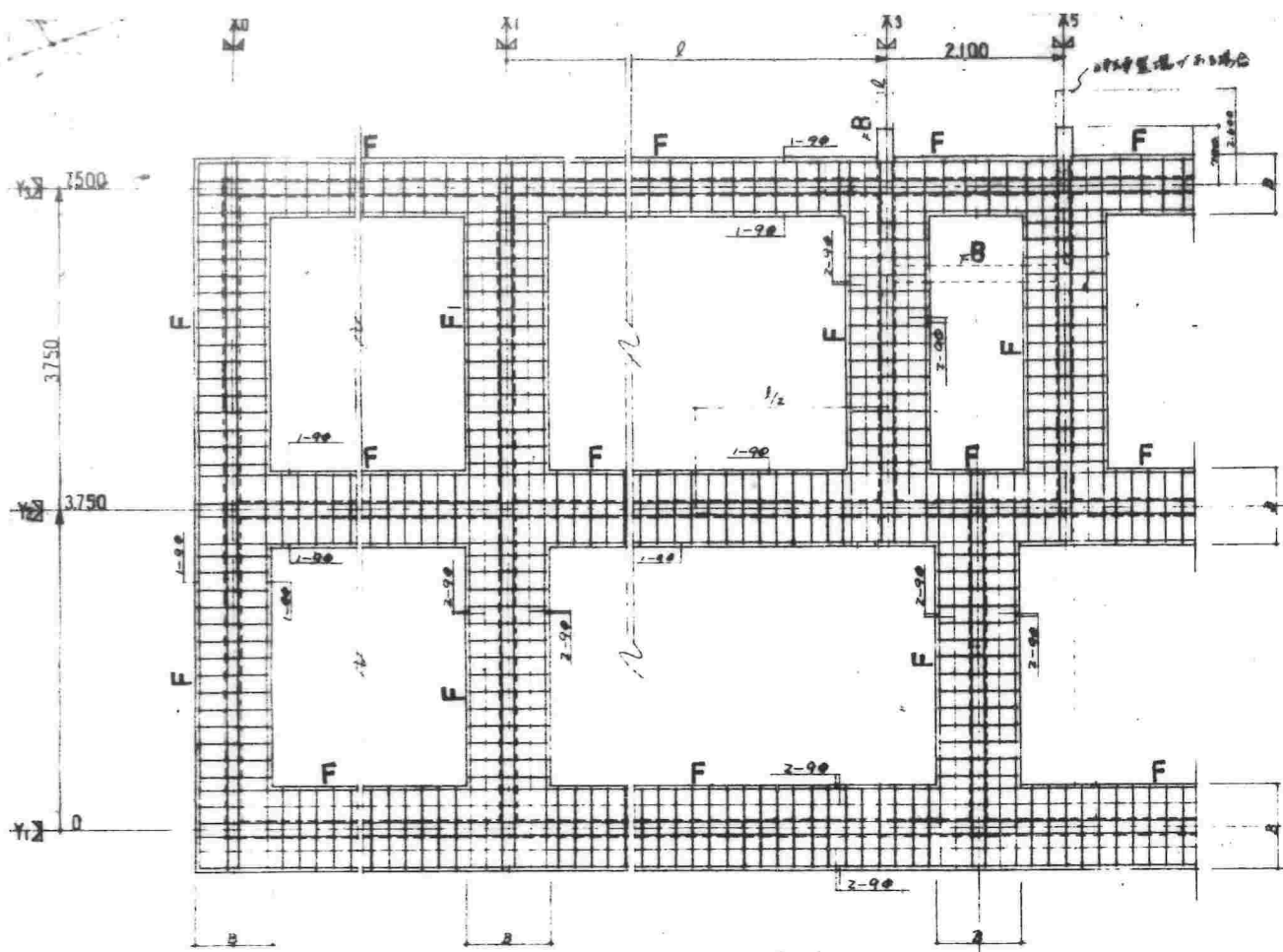
基礎平面詳細図 1:50
