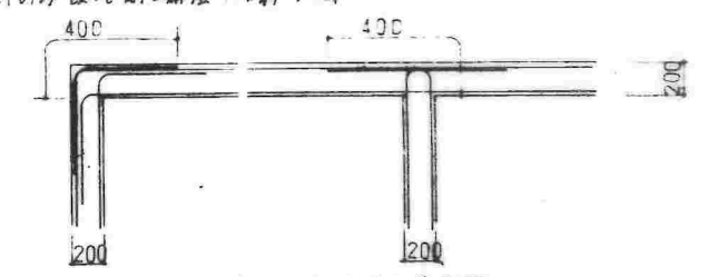
基礎梁上端筋位置要領
