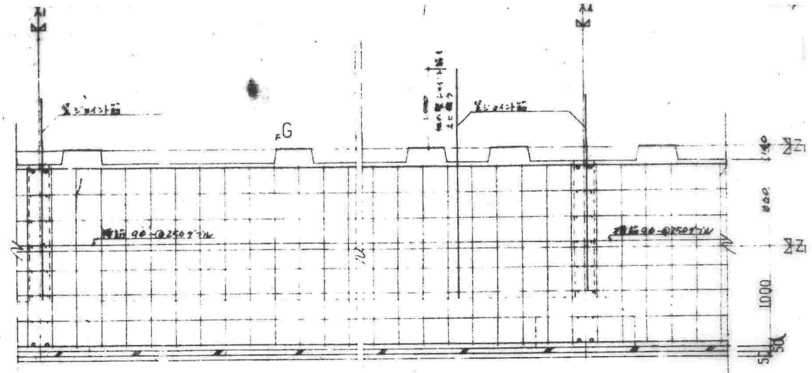
Y1通り基礎梁配筋詳細図 1:30
