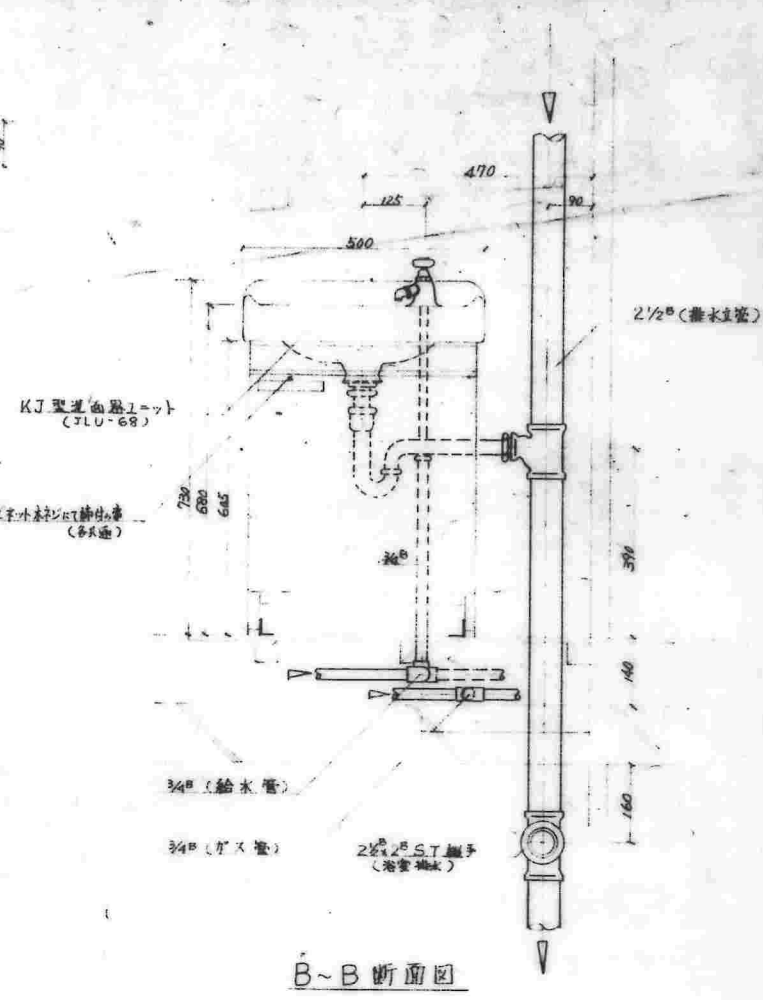
脱衣室廻り配管詳細図 S=1/10
