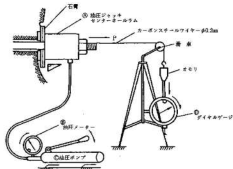
図 4-3 引抜試験概観図
