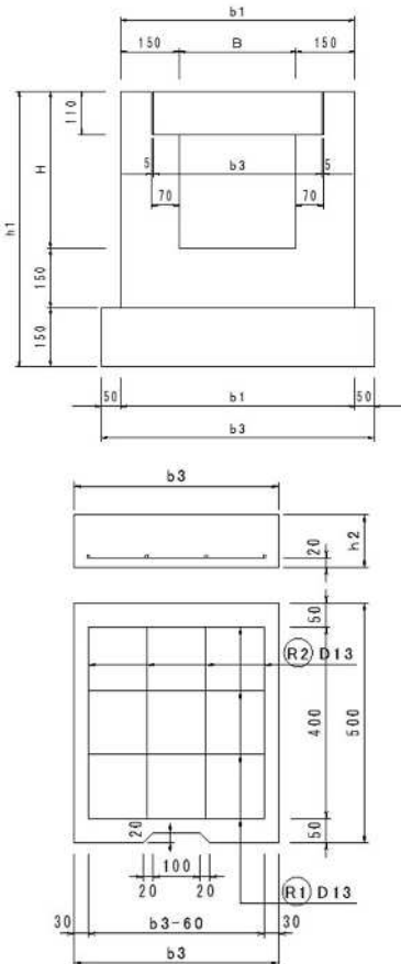
U4型(場所打ちU型側溝:蓋付き)寸法及び材料表
