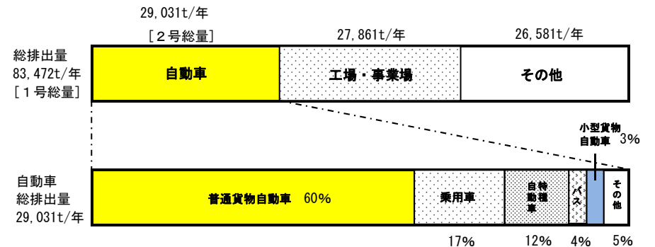
図4-3-1 窒素酸化物排出量 (平成21年度)
