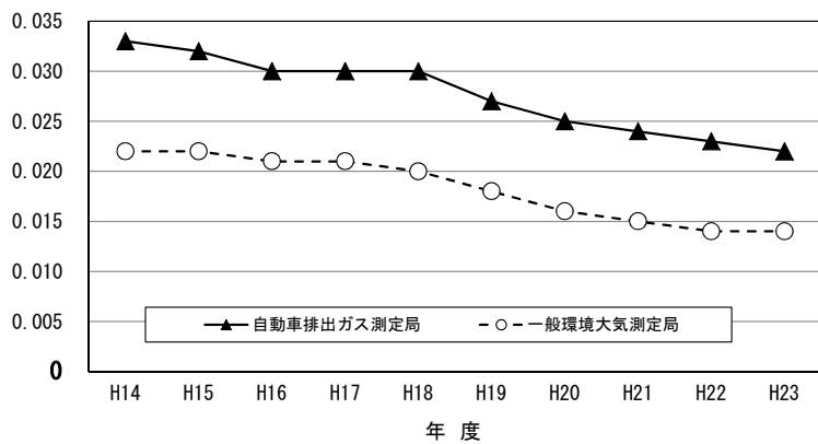
図4-3-3(2) 二酸化窒素濃度の推移(年平均値)
