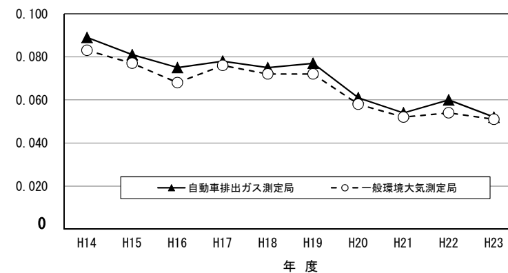
図4-3-3(3) 浮遊粒子状物質濃度の推移(2%除外値)
