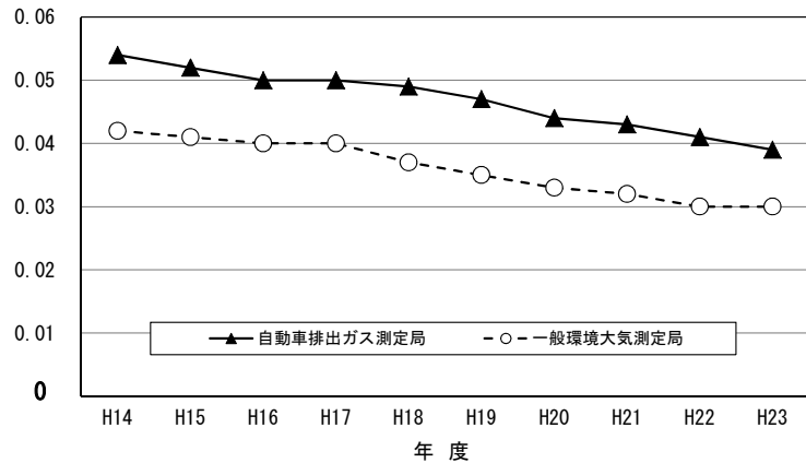
図4-3-3(1) 二酸化窒素濃度の推移(98%値)
