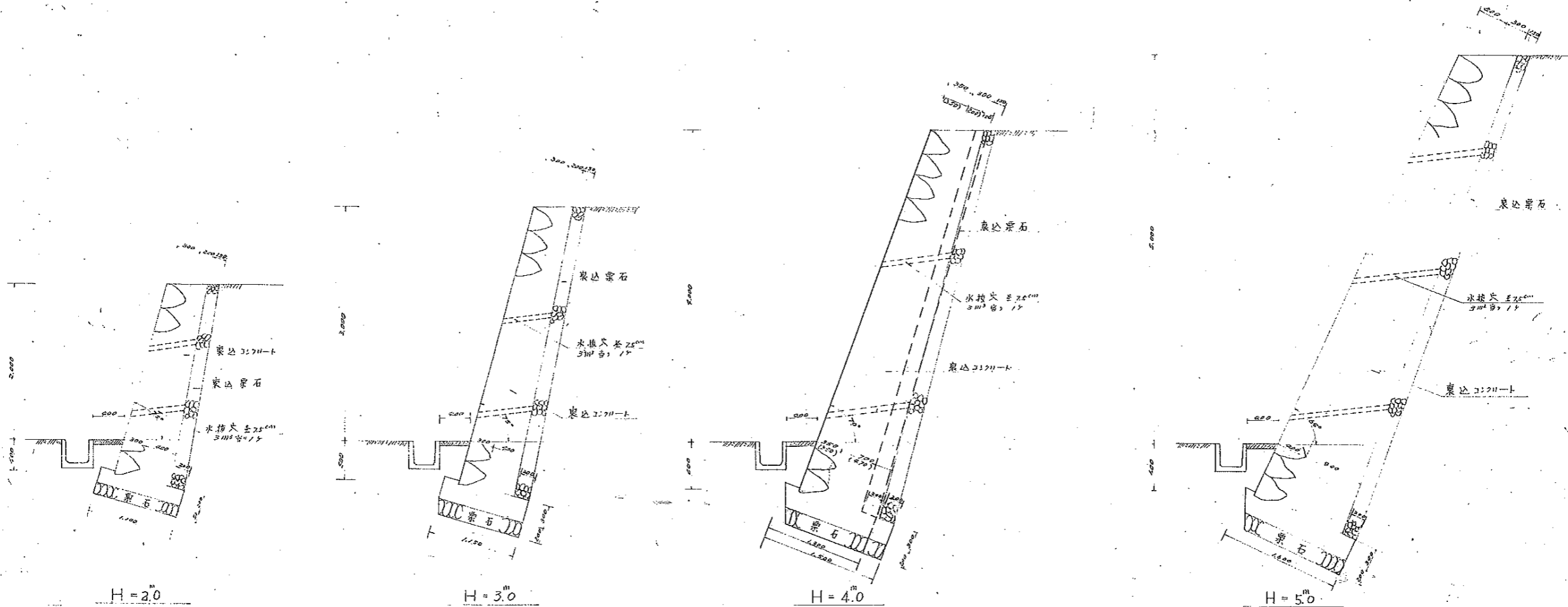
面知石線積れ透擁壁 s=1/50 (註) H=2.0, 3.0, 5.0ハ調査同様, H=4.0ハ切土 場合/( )内ノ数値=スル
