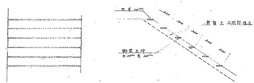
筋芝工詳細図 s=1/50
