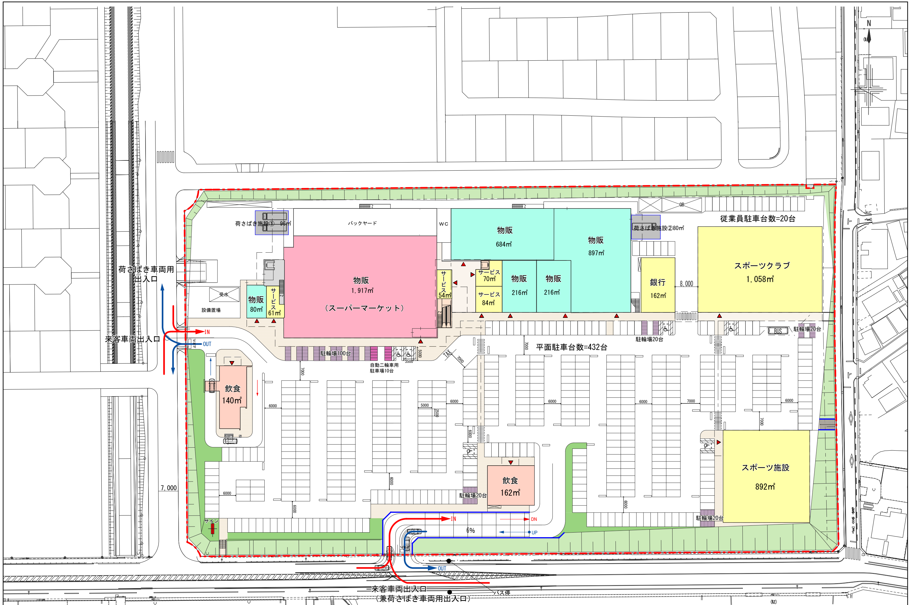
図面3 建物配置図兼1階平面図 (S=1/800)
