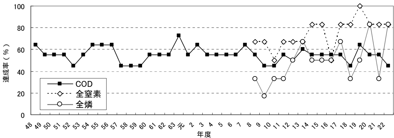
伊勢湾・三河湾における環境基準達成率（COD、全窒素及び全磷）の経年変化
