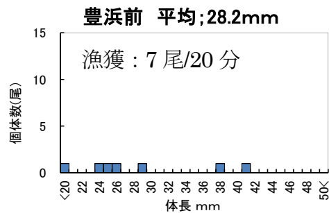
図 3月4日小規模試験びき結果 (イカナゴ仔魚体長組成)
