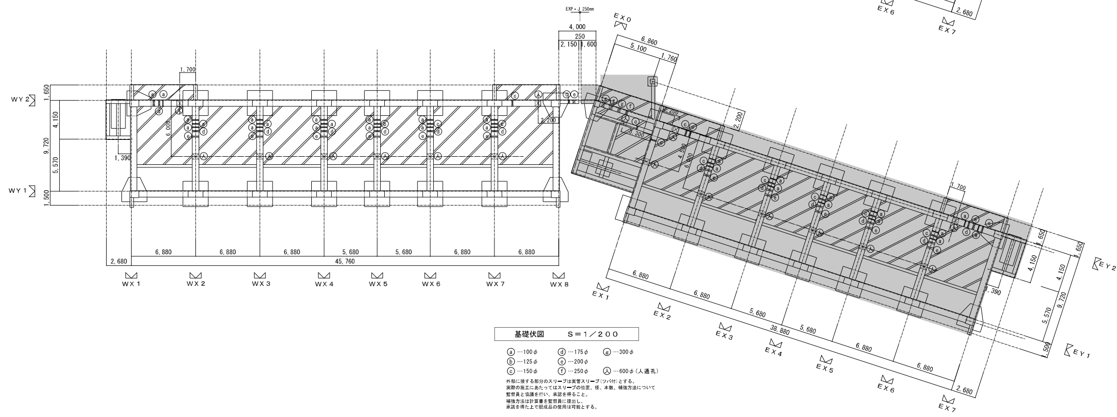
2階～9階伏図 S=1/200
