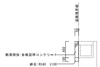
北側道路 側溝補強工復旧詳細図 1/30
