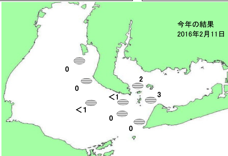
図1 2月11日カイトネット調査結果 ※採集尾数（曳網1分あたり）と体長組成
